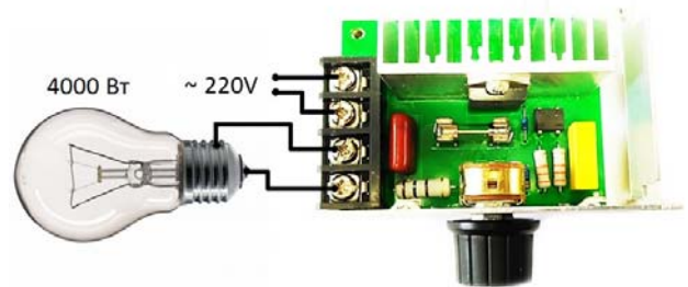
Вид изнутри и схема подключения. Рис. 2
